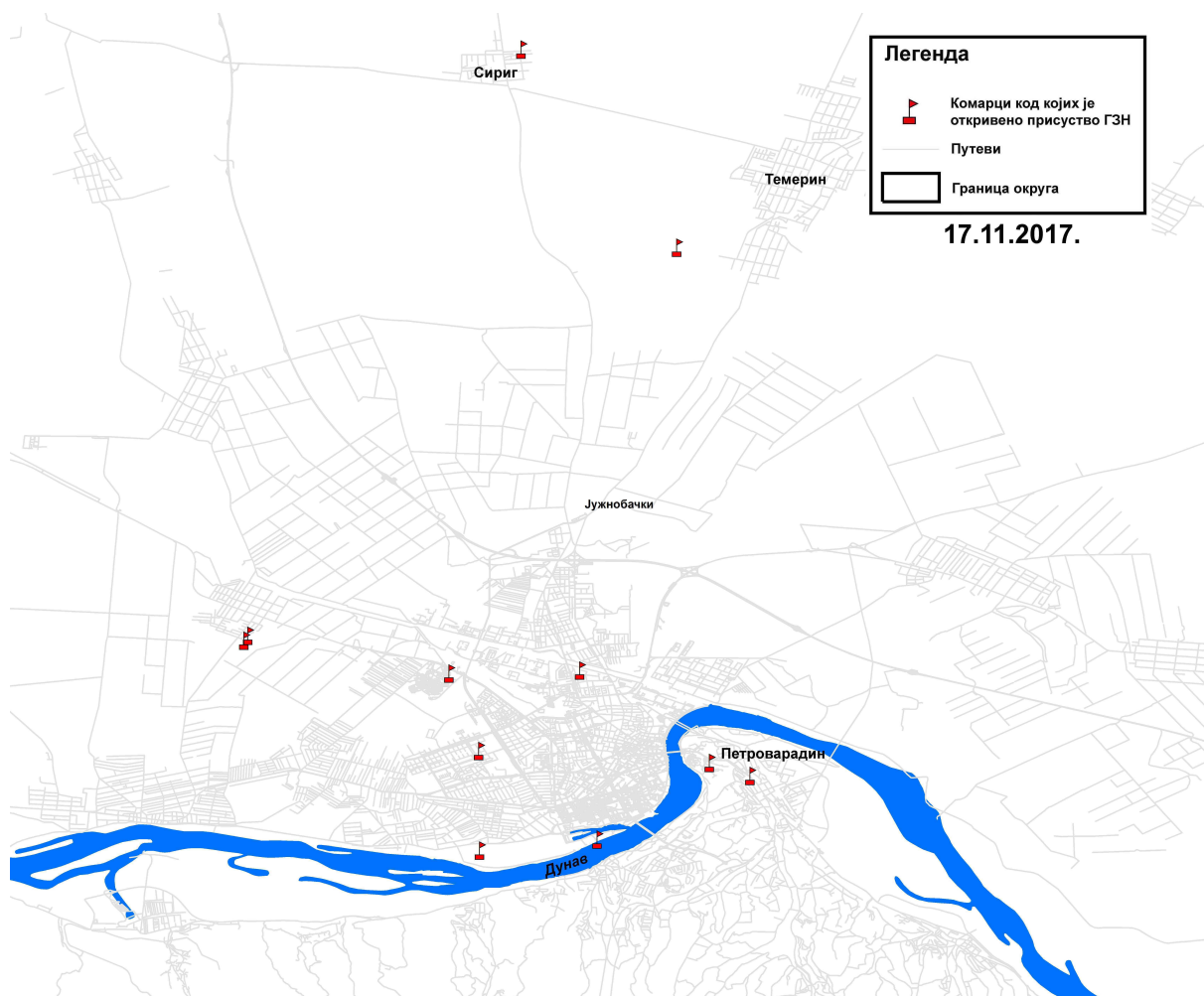
Мапа 3.2. Присуство вируса Западног Нила у узорцима комараца, Град Нови Сад, Темерин и Сириг, сезона надзора 2017. години
