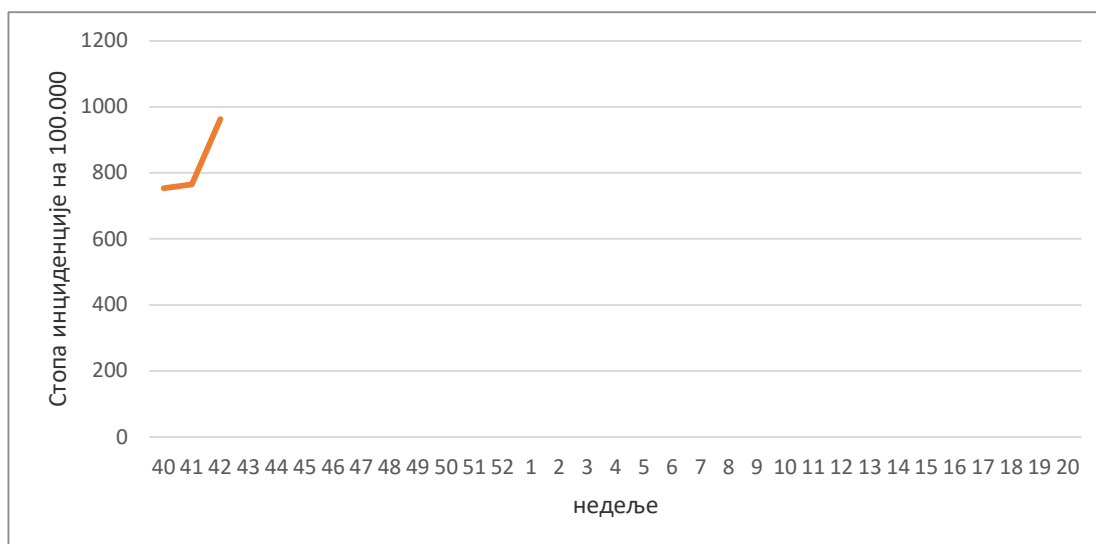
Графикон 3. Стопа инциденције акутних респираторних инфекција, према извештајним недељама у сезони 2020/2021, сентинелни надзор
