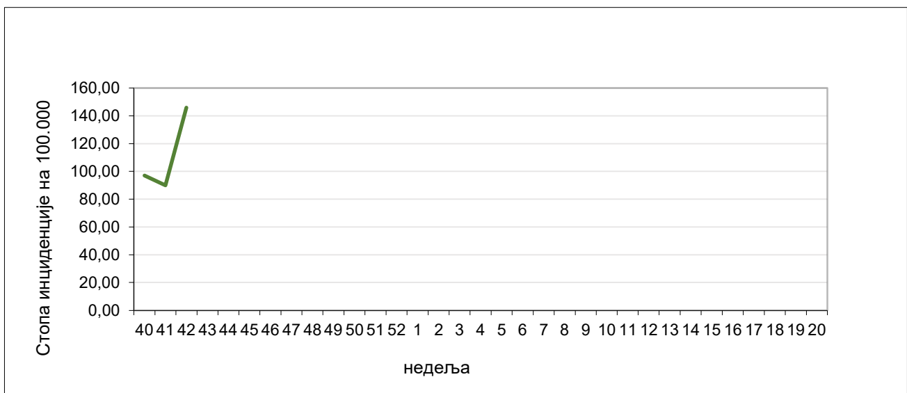
Графикон 2. Стопа инциденције обољења сличних грипу, према извештајним недељама у сезони 2020/2021, сентинелни надзор
