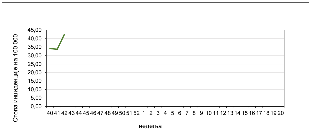
Графикон 1. Стопа инциденције обољења сличних грипу, према извештајним недељама, сезона 2020/2021, популациони надзор
